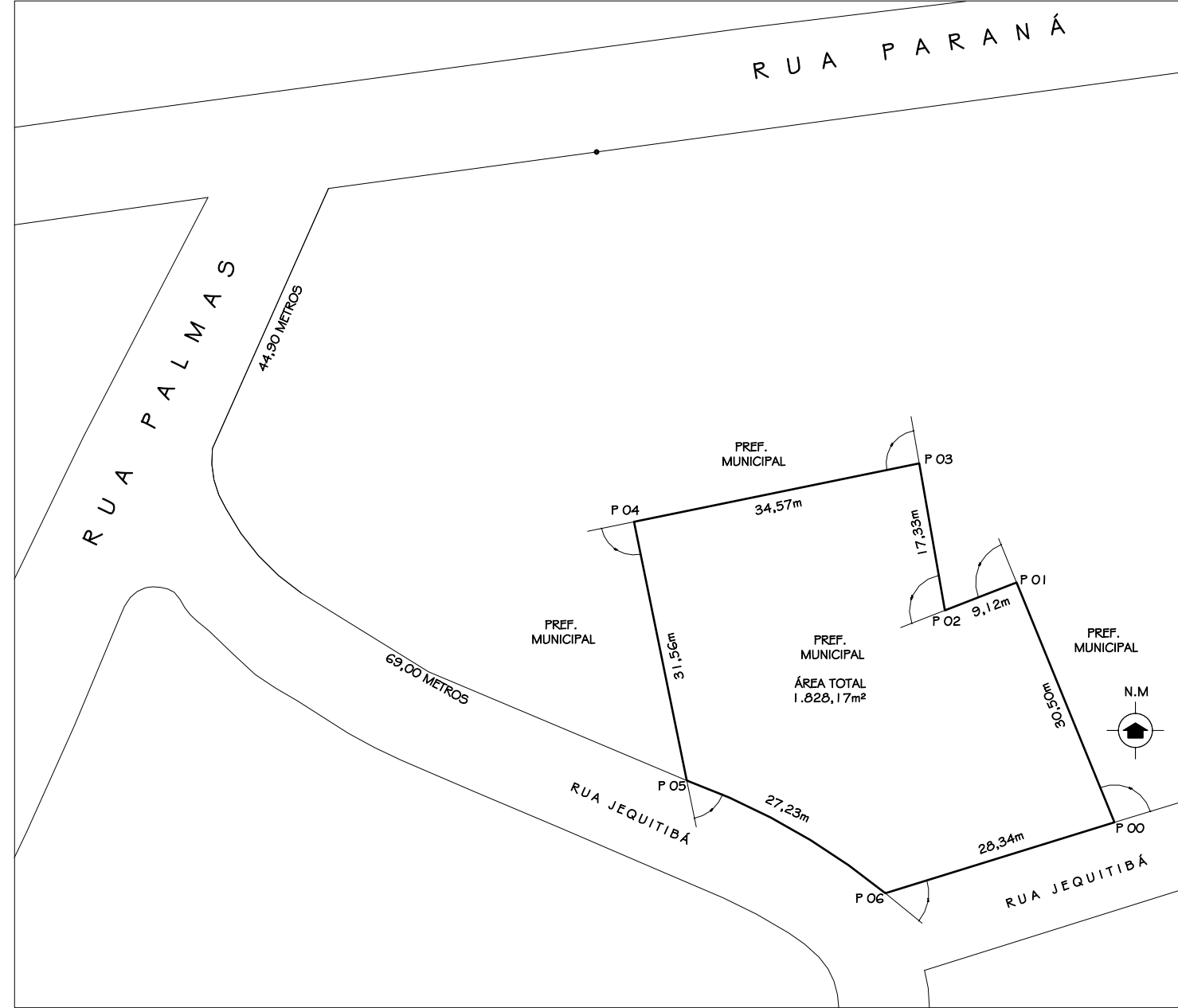
PLANTA DE TERRENO ESCALA:..... 1 / 500
